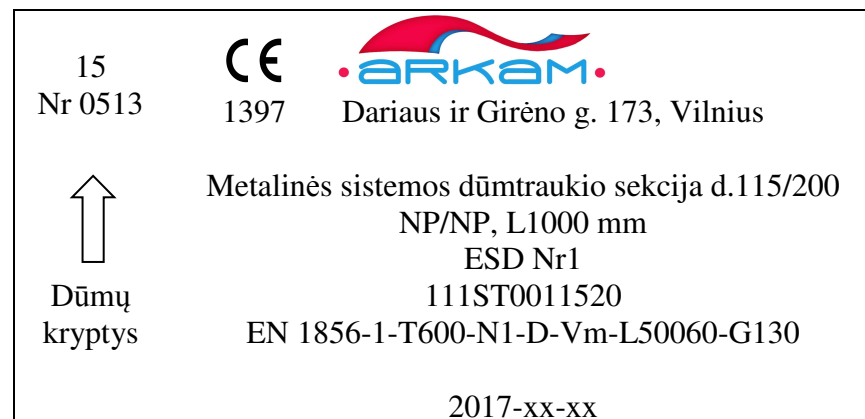
1 pav. Dvisienių dūmtraukių sistemos elementų ženklinimo pavyzdys
