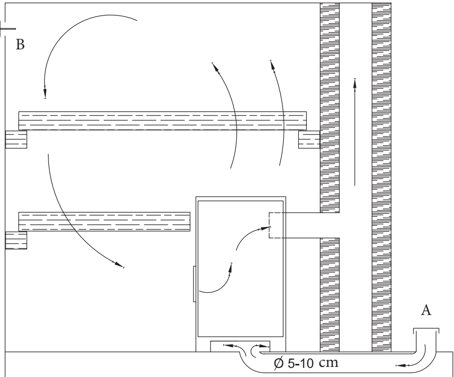
Pav. 1. Natūrali ventiliacija
